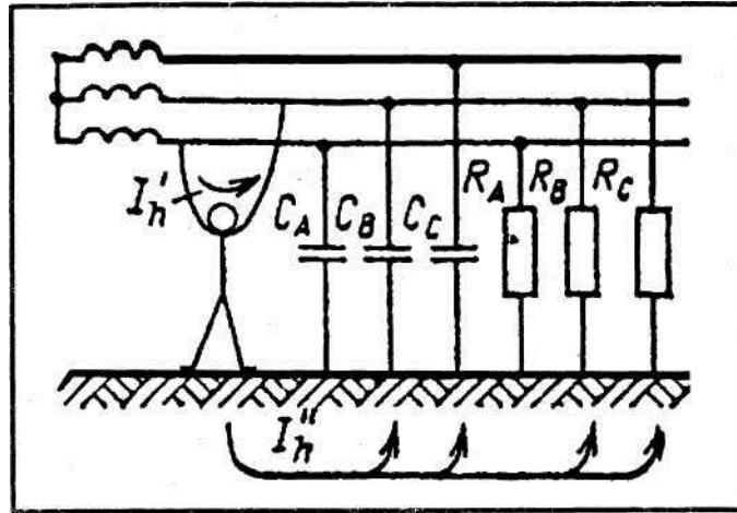
Рис. 18. Двофазне дотикання
