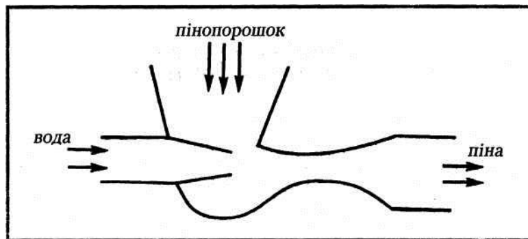
Рис. 12. Схема піногенератора
