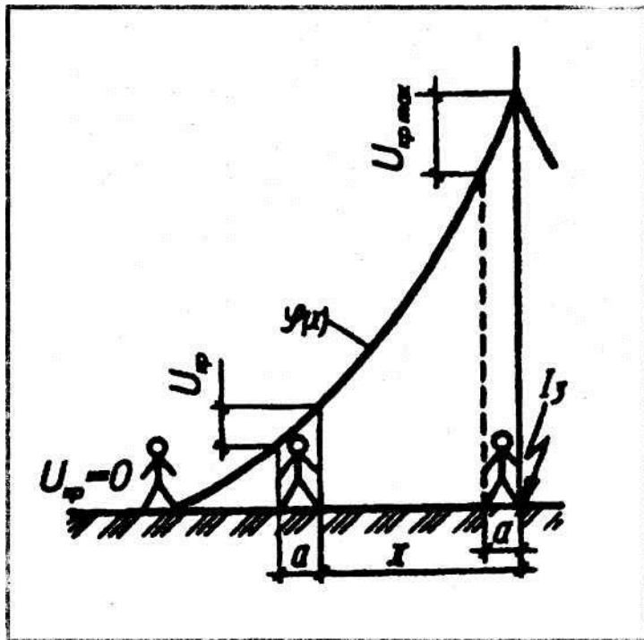
Рис. 19. Дія напруги кроку
