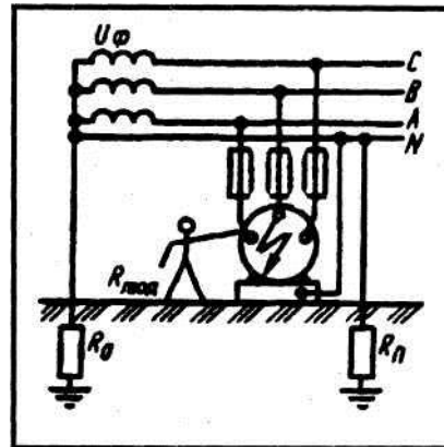
Рис. 26. Занулення
