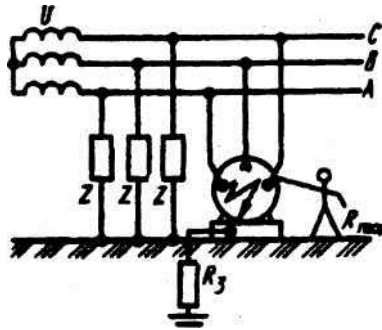
Рис. 25. Заземлення
