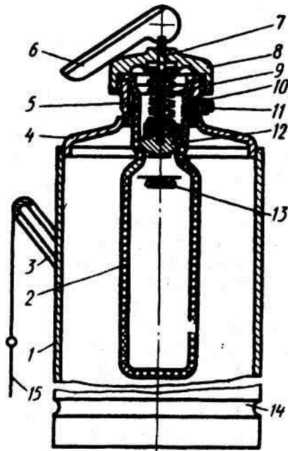
Рис. 13. Вогнегасник ВХП-10: 1 — корпус; 2 — кислотний стакан; 3 — бокова ручка; 4 — перехідник; 5 — горловина; 6 — рукоятка; 7 — шток; 8 — кришка; 9 — пружина; 10 — сприк; 11 — мембрана; 12 — гумовий клапан; 13 — рівень кислотної частини; 14 — дно; 15 — голка
